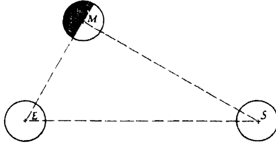
من كتاب أريستارخوس في حجوم وأبعاد الشمس والقمر. الشكل الأعلى: الفرقان القمري. الشكل الأسفل: رسمٌ تخطيطي للخسوف القمري.
